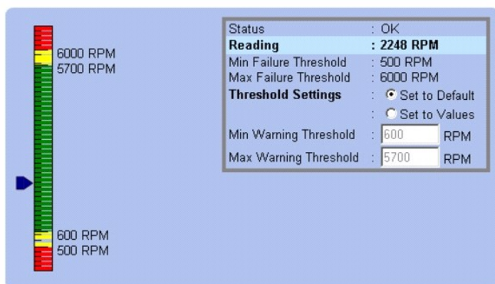
Abbildung 5-2. Messanzeige
